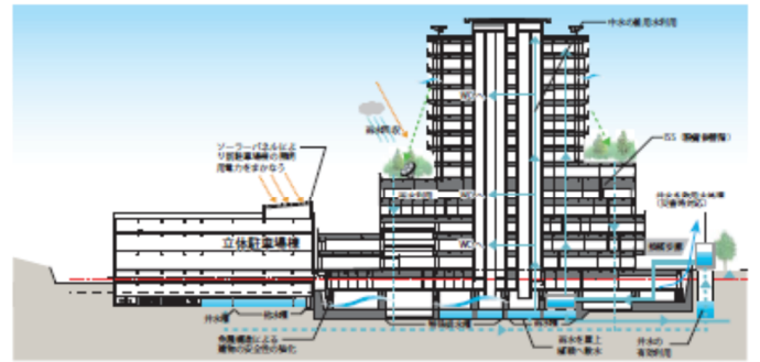
▲環境計画(断面図)
