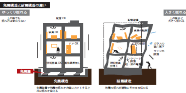
図1 免震構造設置
