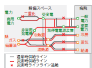
図2 供給ラインの二重化
